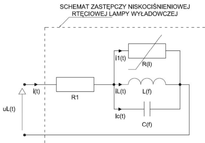
Rys. 4. Schemat zastępczy niskociśnieniowej rtęciowej lampy wyładowczej.
