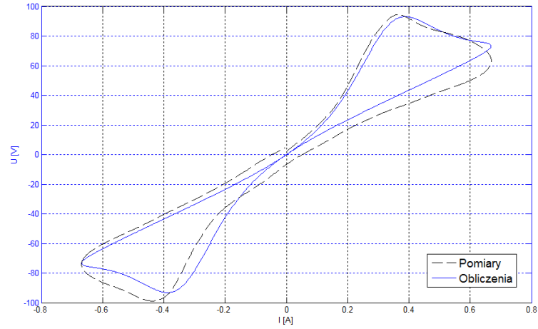
Rys. 8. Napięcie u(t) na lampie dla częstotliwości 500Hz dla badań modelowych oraz badań empirycznych
