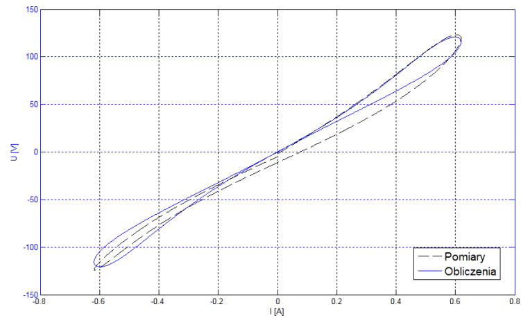
Rys. 9. Napięcie u(t) na lampie dla częstotliwości 10kHz dla badań modelowych oraz badań empirycznych
