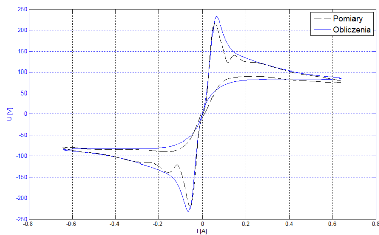
Rys. 7. Napięcie u(t) na lampie dla częstotliwości 50Hz dla badań modelowych oraz badań empirycznych
