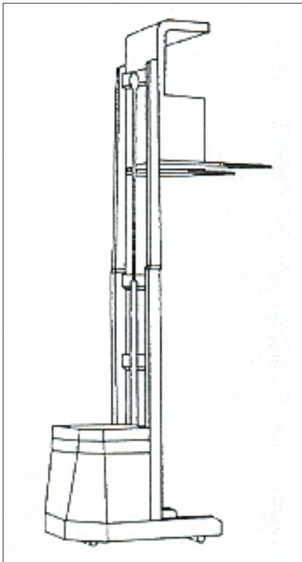
Rys. 7. Wózek podnośnikowy z operatorem podnoszonym wraz z ładunkiem (ang. truck with elevatable operating position). Źródło: PN-ISO 5053: 1999.
