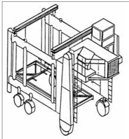
Rys. 10. Wózek podnośnikowy bramowy (ang. stacking high-lift straddle carrier). Źródło: PN-ISO 5053: 1999.
